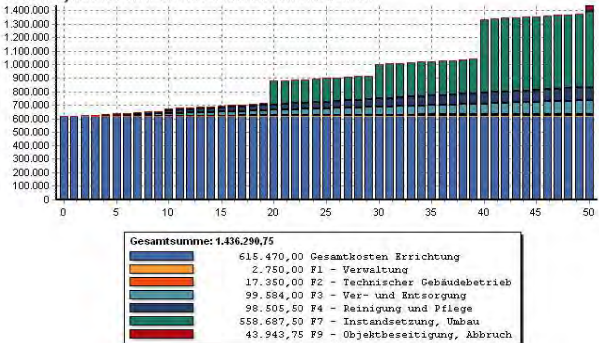
Abb. 12: Verlauf der Lebenszykluskosten von Haus K nach Kosten und Jahren nach statischer Bewertung mit der Software ABK.
